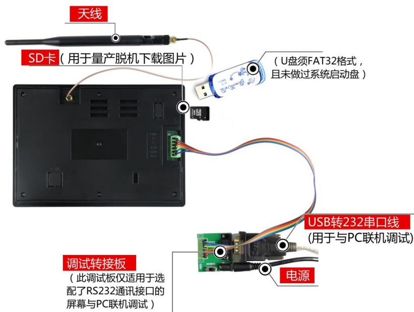
图 1-3 RS232 调试工具图
