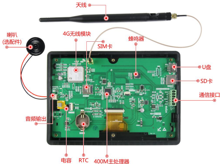
图 1-2 硬件配置图
